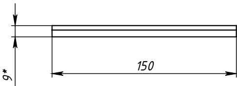
Поз.4 (Накладка)
