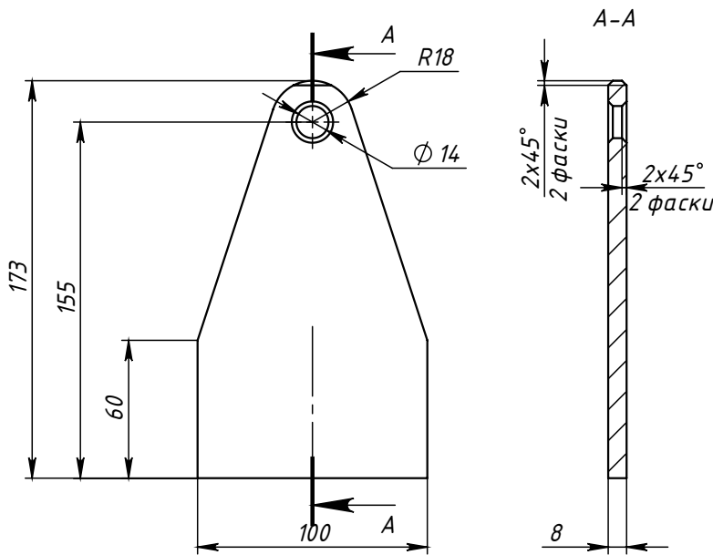
Поз.3 (Проушина)
