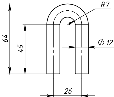
Поз.2 (Ушко) 1:2
